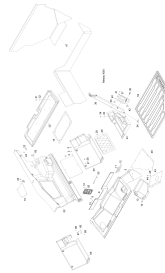
Verkleidungsteile
