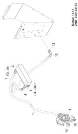
Wärmetauscher Leitungen Lüftermotor
