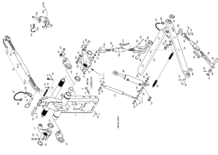
Hubwerk hinten
