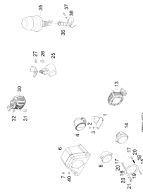
Zusatzbeleuchtung
