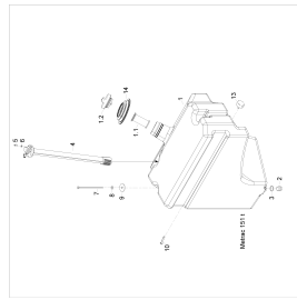
Kraftstofftank
