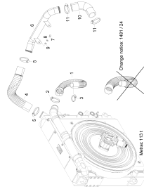
Leitungen Ladeluftkühler Metrac H95
