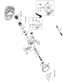
Zapfwelle vorne
