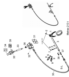
Schaltung S-L
