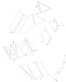
Schwermatten
