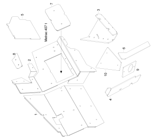
Dämmmatten
