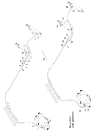
Hydraulikleitungen für Hubwerk hinten
